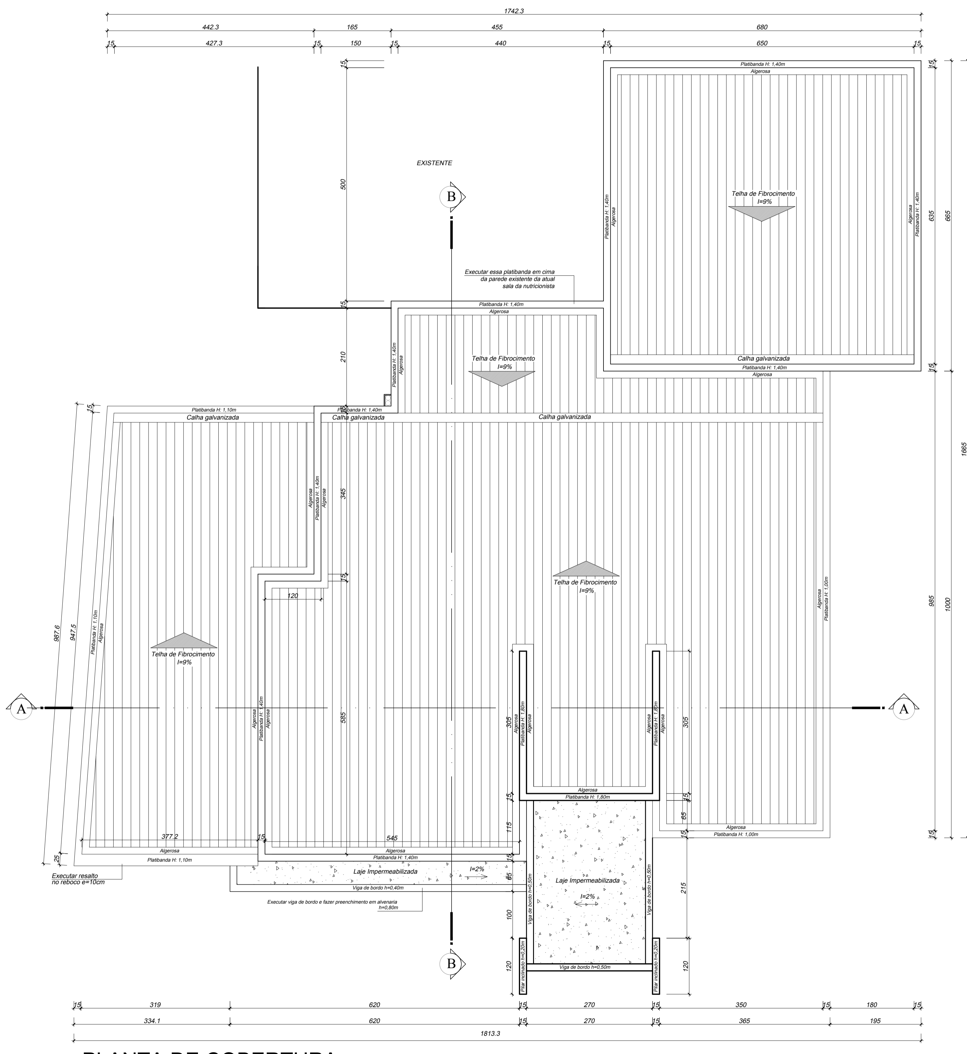
PLANTA DE COBERTURA ESC. 1/50
