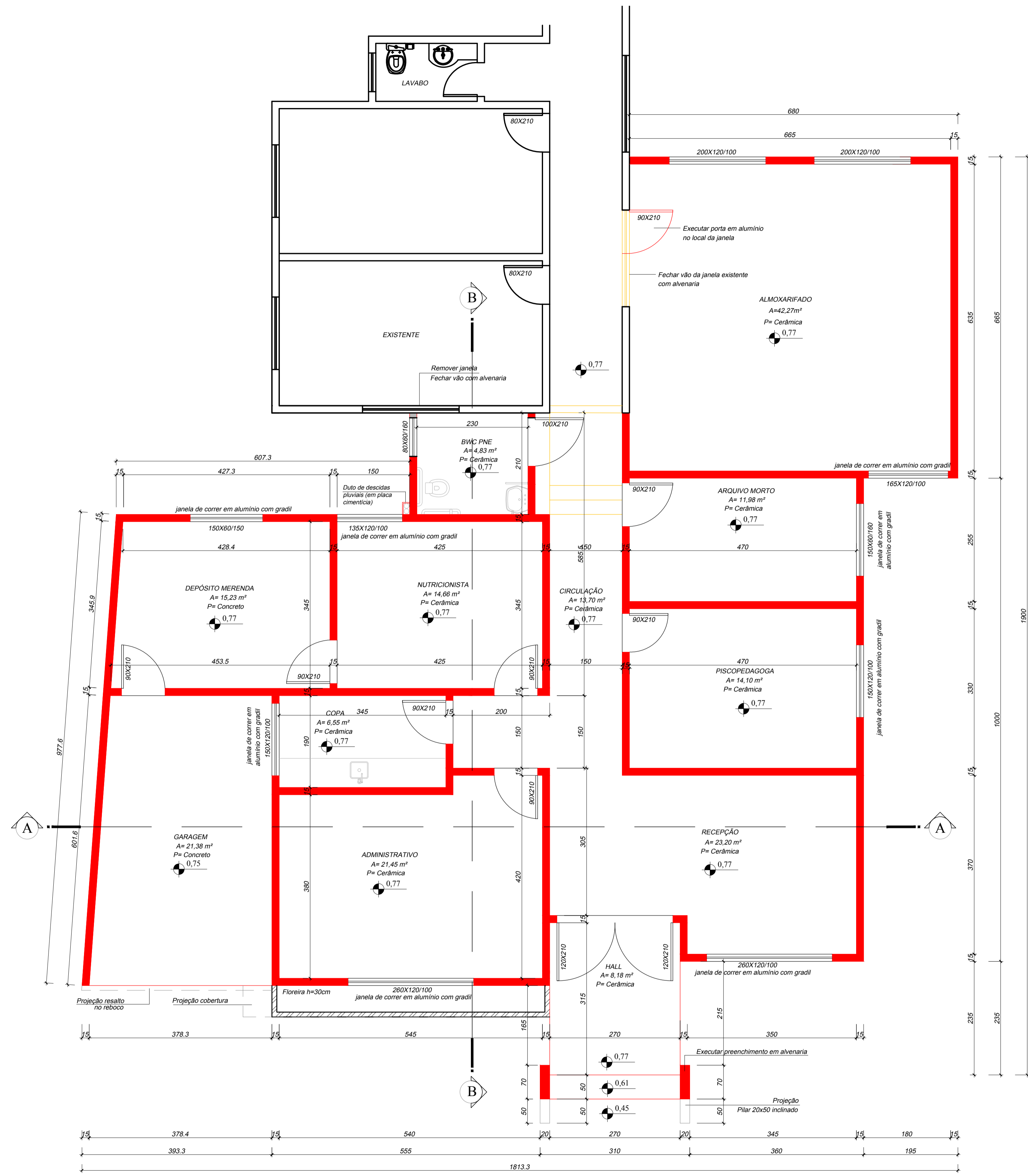
PLANTA BAIXA ESC. 1/50 ÁREA TOTAL= 217,45m²
