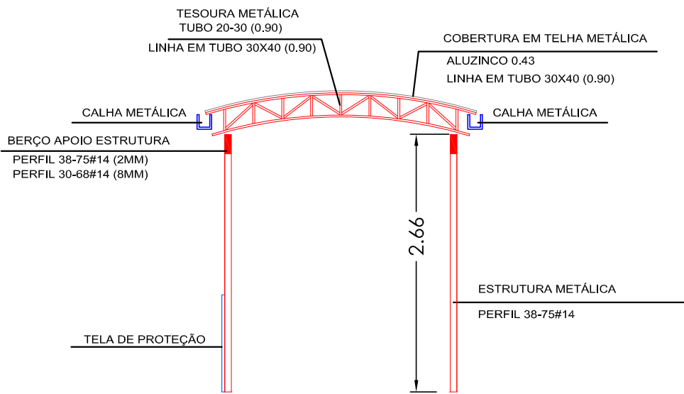
CORTE ESQUEMÁTICO
