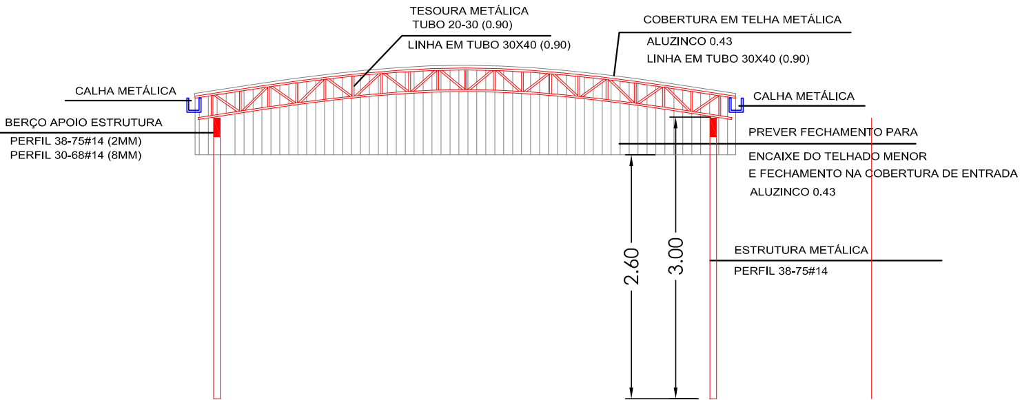
CORTE ESQUEMÁTICO
