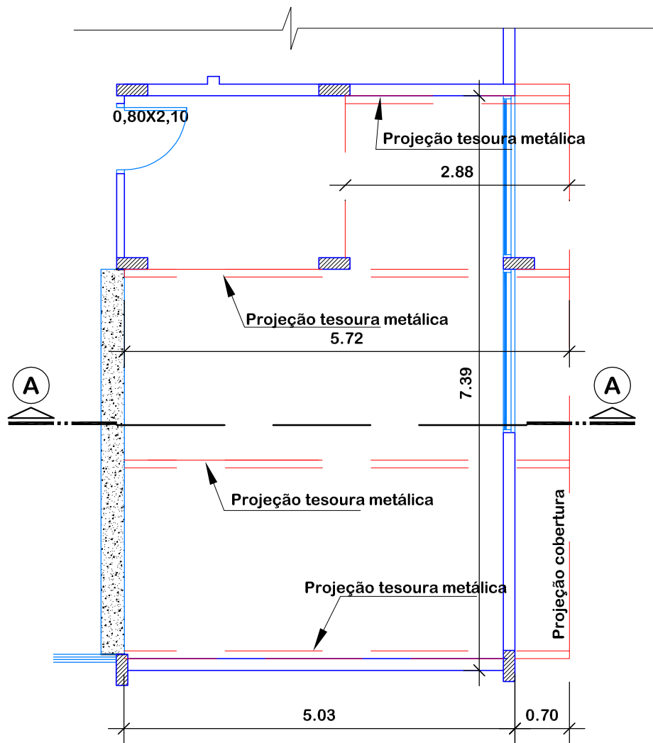
PLANTA BAIXA
