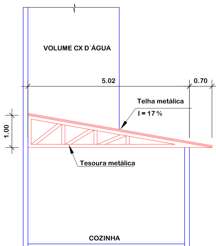
CORTE AA
