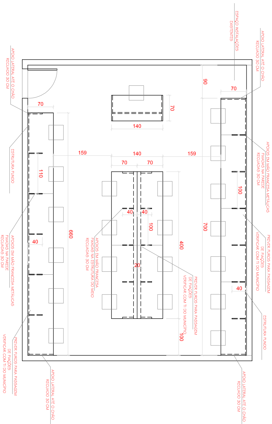
PLANTA BAIXA - MÓVEIS LABORATÓRIO DE INFORMÁTICA Escala: 1/50
