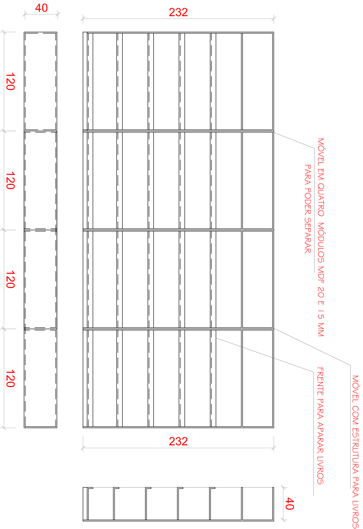
DETALHE 03 - PRATELEIRAS PAREDE Escala: 5/e
