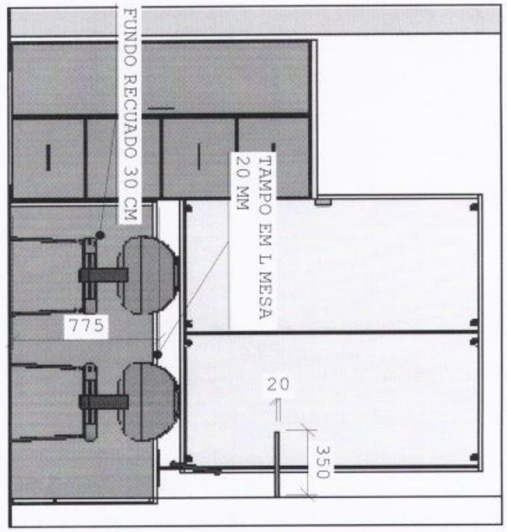
VISTA A 1:25
